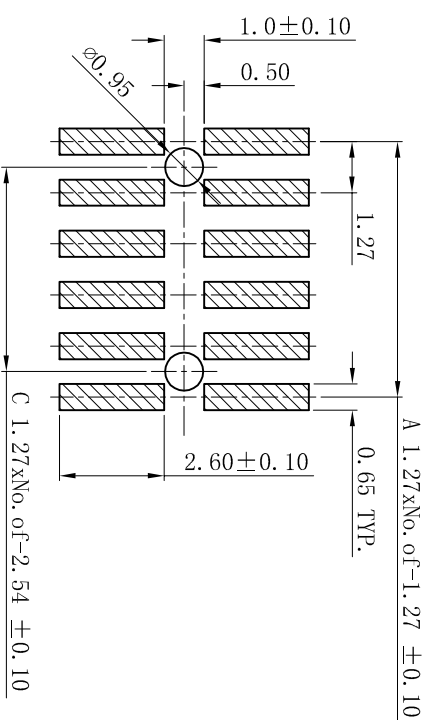
P.C.B LAYOUT: TOP VIEW TOLERANCE: \pm 0.05\text{mm}
