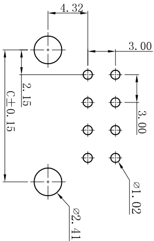
P. C. B. LAYOUT
