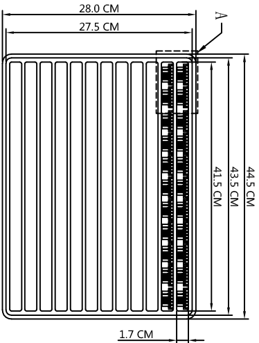
吸塑盘下盖(12格)
