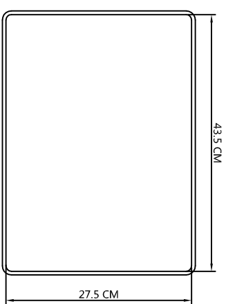
吸塑盘上盖
