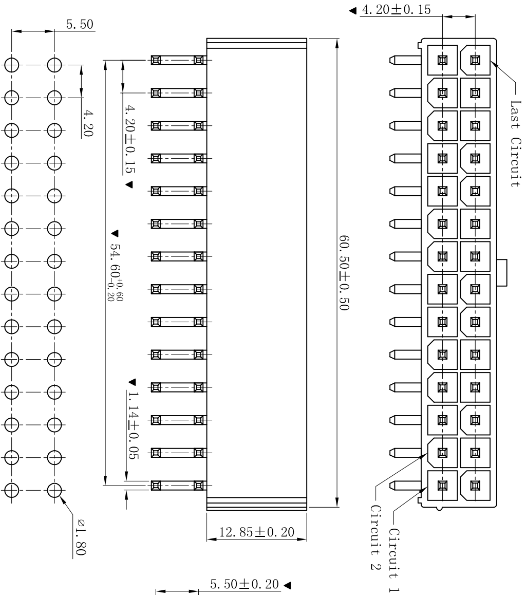
P.C.B LAYOUT
