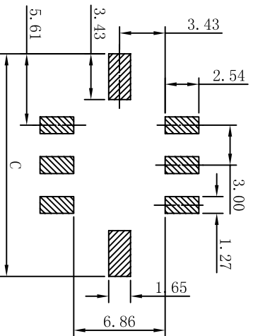
P. C. B. LAYOUT
