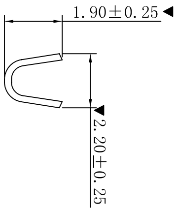
SEC:B-B
